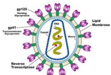
HIV
