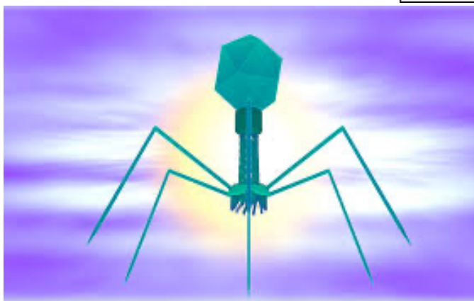
BATTERIOFAGO T2
